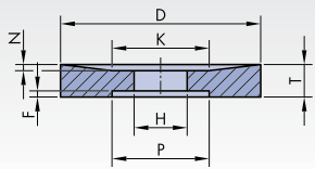
22 D/KxT/NxH-PxF
