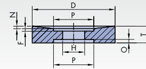
24 DxT/NxH-PxF/G
