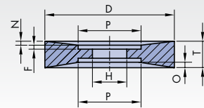
26 DxT/NxH-PxF/G
