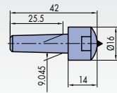
K106 ZYLINDER
