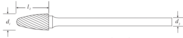
Tree Shape Radius End Forma de árbol Con radio Forme d'ogive Bout hémisphérique
